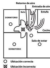
Figure 6: UBICACIONES RECOMENDADAS DE DETECTORES DE HUMO PARA EVITAR CORRIENTES DE AIRE CON PARTICULAS DE COMBUSTIÓN
