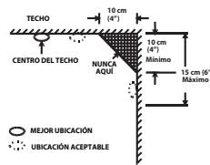
Figure 4: LAS MEJORES Y MÁS ACEPTABLES UBICACIONES RECOMENDADAS PARA INSTALAR DETECTORES DE HUMO
