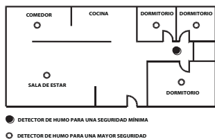
Figure 1: DÓNDE INSTALAR DETECTORES DE HUMO EN UNA VIVIENDA ÚNICA CON SOLO UN DORMITORIO
